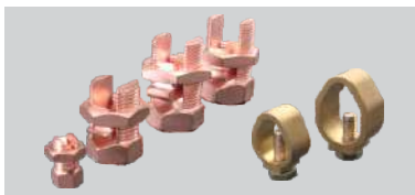
Conector Split y Bolt Conector AB de Bronce
